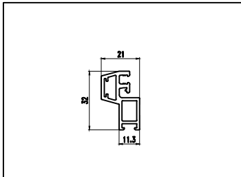
型号: GR90C05 名称: 纱扇 壁厚: 1.60 mm 重量: 0.529 kg/m
