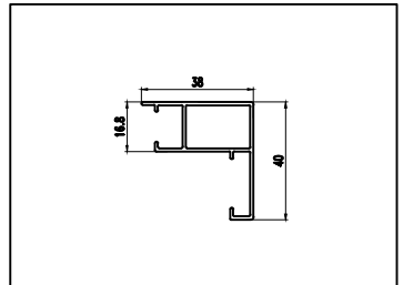
型号: GR90C08 名称: 固定压线框 壁厚: 1.10 mm 重量: 0.149 kg/m
