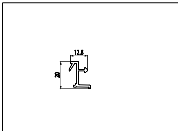
型号: GR90C09 名称: 固定横压座 壁厚: 1.50 mm 重量: 0.198 kg/m
