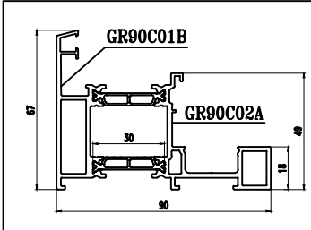
型号: GR90C02 名称: 外框 壁厚: 1.80 mm 重量: 1.886 kg/m
