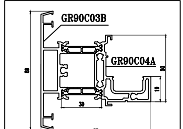
型号: GR90C04 名称: 中挺 壁厚: 1.80 mm 重量: 2.315 kg/m
