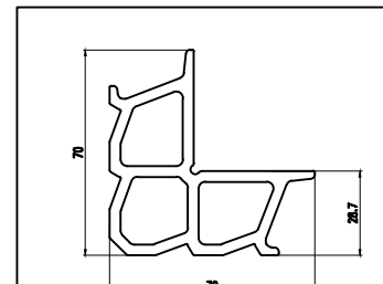
型号: KSYC8017 名称: 角码 壁厚: 3.70 mm 重量: 2.818 kg/m
