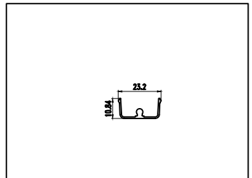
型号: GR90C12 名称: 下滑轨 壁厚: 0.80 mm 重量: 0.128 kg/m
