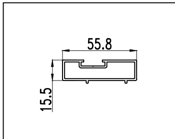
型号: ZDM58A06 名称: 外框收口 壁厚: 1.50 mm 重量: 0.622 kg/m
