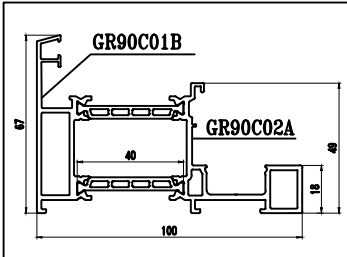
型号: GR90C14 名称: 外框 壁厚: 1.80 mm 重量: 2.036 kg/m
