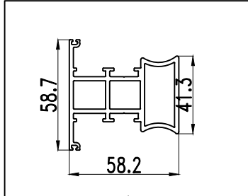
型号: ZDM58A02 名称: 中柱 壁厚: 2.20 mm 重量: 1.734 kg/m
