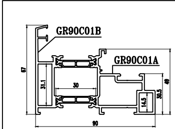
型号: GR90C01 名称: 外框 壁厚: 1.80 mm 重量: 2.052 kg/m
