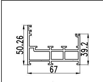
型号: ZDM58A01 名称: 外框 壁厚: 2.20 mm 重量: 1.593 kg/m
