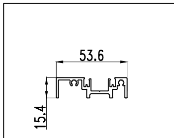
型号: ZDM58A12 名称: 下轨辅料 壁厚: 1.60 mm 重量: 0.678 kg/m
