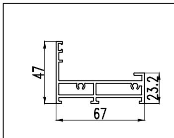
型号: ZDM58A11 名称: 下框料 壁厚: 2.00 mm 重量: 1.342 kg/m
