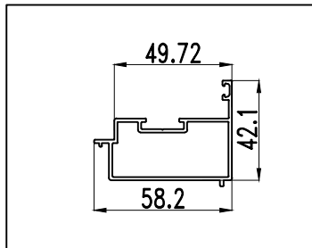
型号: ZDM58A07 名称: 外框收口 壁厚: 1.40 mm 重量: 0.751 kg/m
