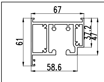
型号: ZDM58A10 名称: 上吊轨 壁厚: 2.00 mm 重量: 2.322 kg/m
