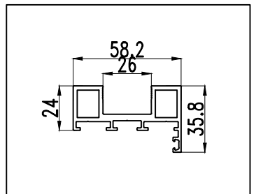
型号: ZDM58A13 名称: 横扇料 壁厚: 2.20 mm 重量: 1.213 kg/m
