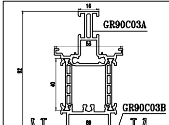
型号: GR90C15 名称: 中挺 壁厚: 1.80 mm 重量: 2.339 kg/m
