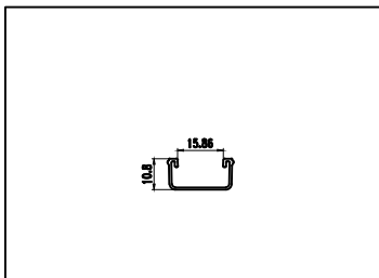
型号: KSYC8012 名称: 上滑轨 壁厚: 0.80 mm 重量: 0.114 kg/m
