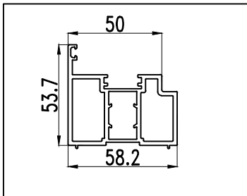
型号: ZDM58A05 名称: 收口 壁厚: 2.20 mm 重量: 1.613 kg/m
