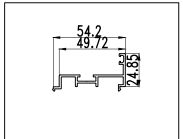
型号: ZDM58A08 名称: 收口 壁厚: 1.50 mm 重量: 0.489 kg/m
