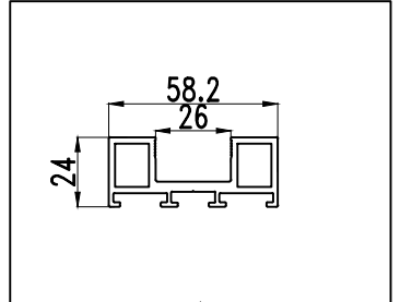
型号: ZDM58A04 名称: 扇料 壁厚: 2.20 mm 重量: 1.141 kg/m
