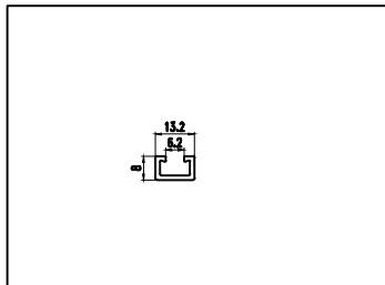
型号: GR90C11 名称: 传动杆(氧化黑) 壁厚: 1.50 mm 重量: 0.125 kg/m
