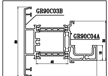
型号: GR90C16 名称: 中挺 壁厚: 1.60 mm 重量: 2.465 kg/m
