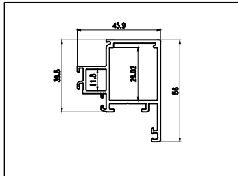
型号: GR90C07 名称: 扇料 壁厚: 1.80 mm 重量: 1.024 kg/m
