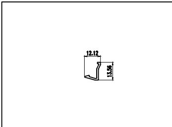
型号: GR90C06 名称: 纱扇压线 壁厚: 1.30 mm 重量: 0.088 kg/m
