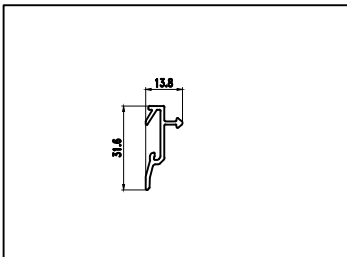
型号: GR90C10 名称: 固定压线座 壁厚: 1.50 mm 重量: 0.226 kg/m
