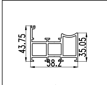
型号: ZDM58A03 名称: 半中柱 壁厚: 2.20 mm 重量: 1.523 kg/m
