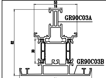
型号: GR90C03 名称: 中挺 壁厚: 1.80 mm 重量: 2.189 kg/m
